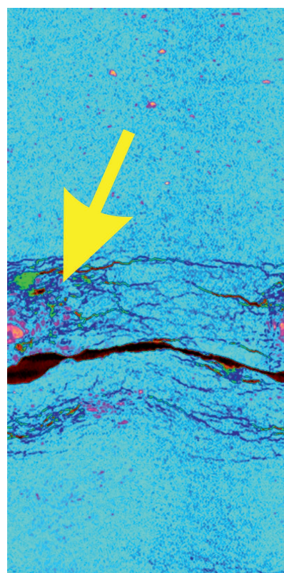
Rys. 24. Przykład obrazu tomografii rentgenowskiej (CT) silnie zmienionych utworów ognia \text{Na}_2
