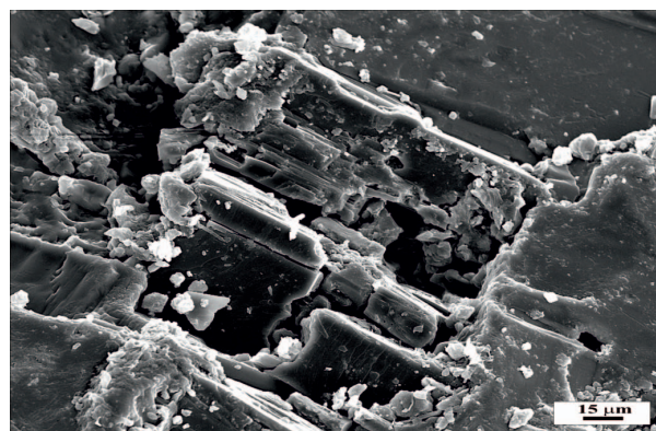
Rys. 7. Tabliczkowe kryształy anhydrytu tkwiące pomiędzy kryształami halitu (obraz SEM)
