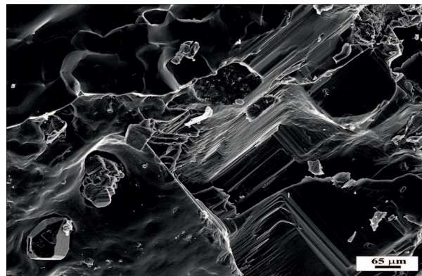
Rys. 6. Kryształy halitu grubokrystalicznego wraz z polewami halitowymi (obraz SEM)
