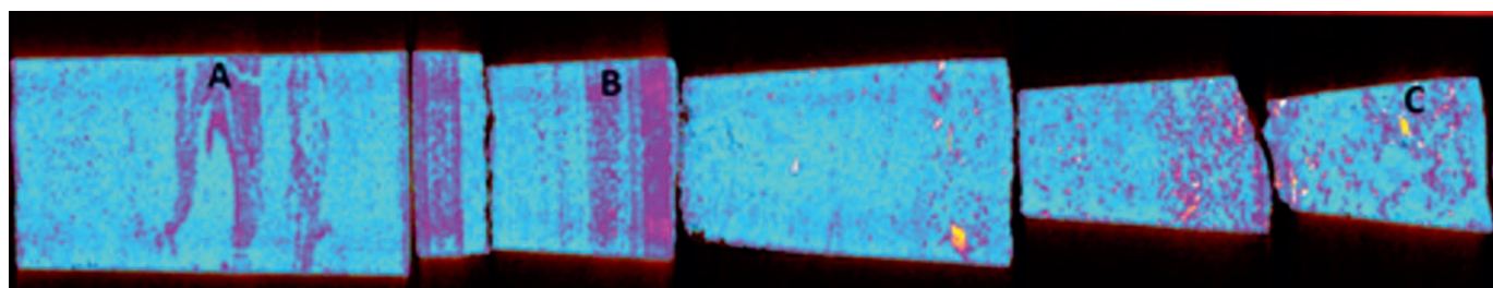
Rys. 3. Sole dolnomioceńskie w obrazie tomograficznym (CT), na którym widoczne są odkształcenia plastyczne wkładek iłasto-mułowcowych (A), laminacja równoległa (B), strefa brekcji solnej (C)
