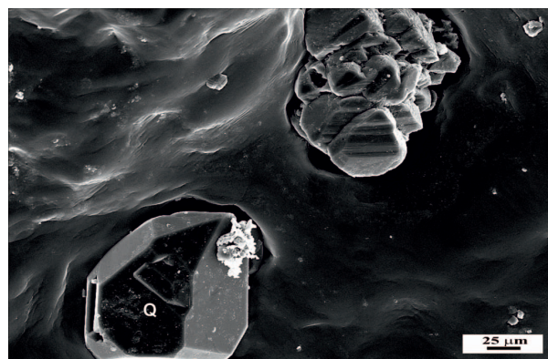
Rys. 8. Ziarno kwarcu terygenicznego (Q) tkwiące na powierzchni pokrywy halitowej (obraz SEM)
