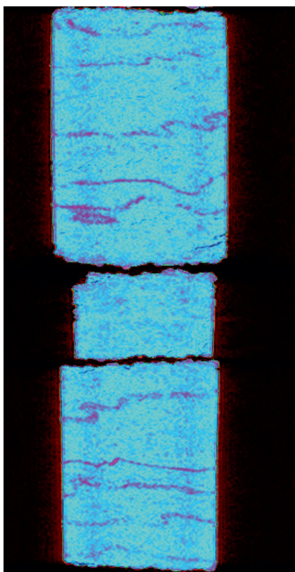
Rys. 5. Plastyczna deformacja lamin ilastych występujących w obrębie soli kamiennej (obraz tomograficzny CT)
